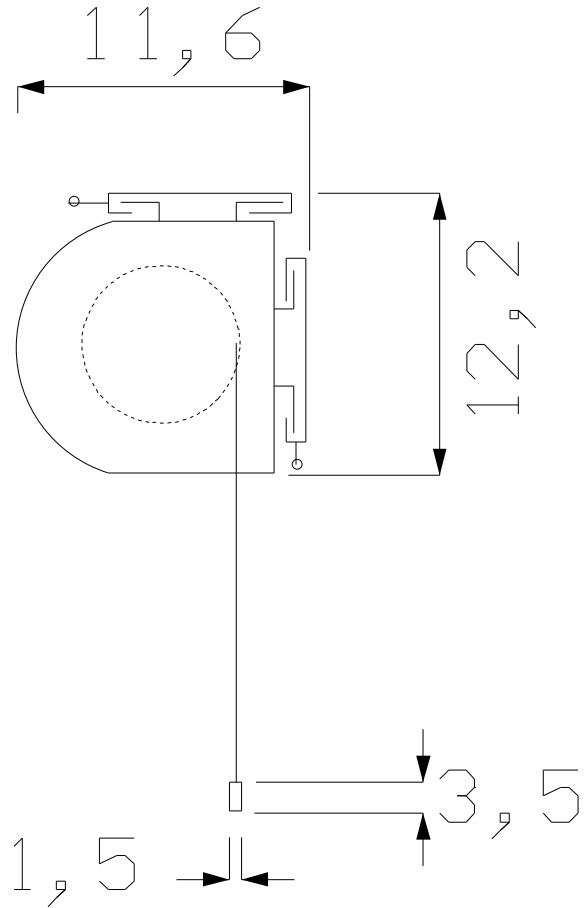
SEZIONE CASSONETTO
